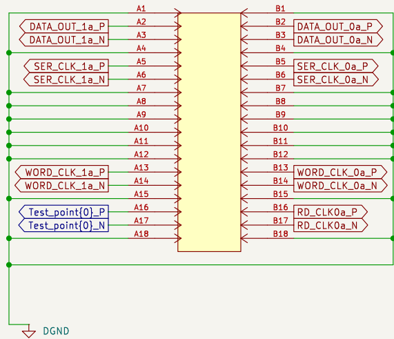
J1 CONN_MINI_SAS_RCPT_36POS_SLD_SMD 757840140:CONN36_B4-0140_MOL
