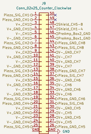
DB50 piezo connector
