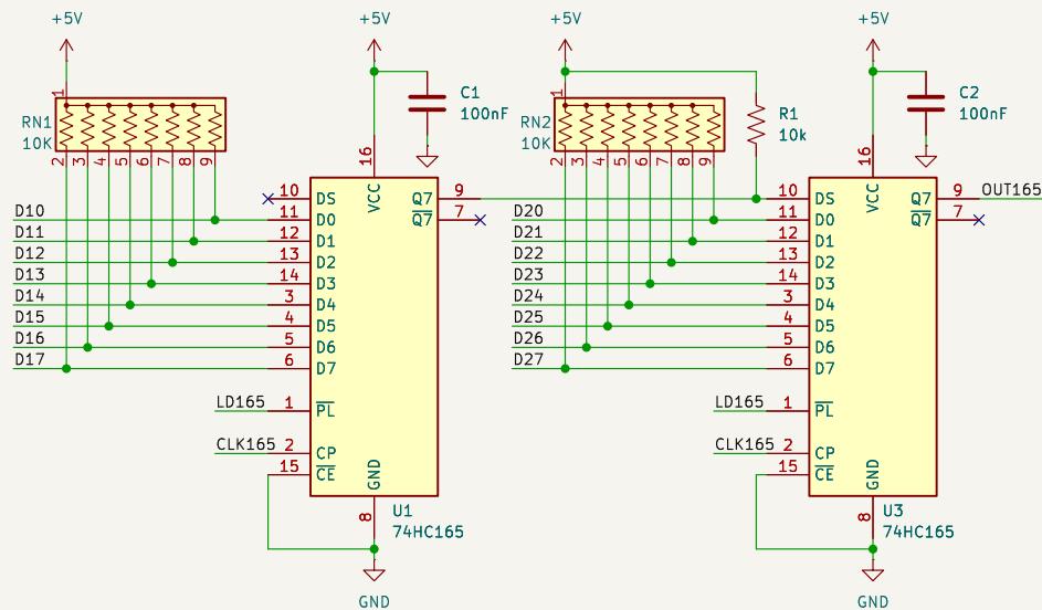
74HC165
