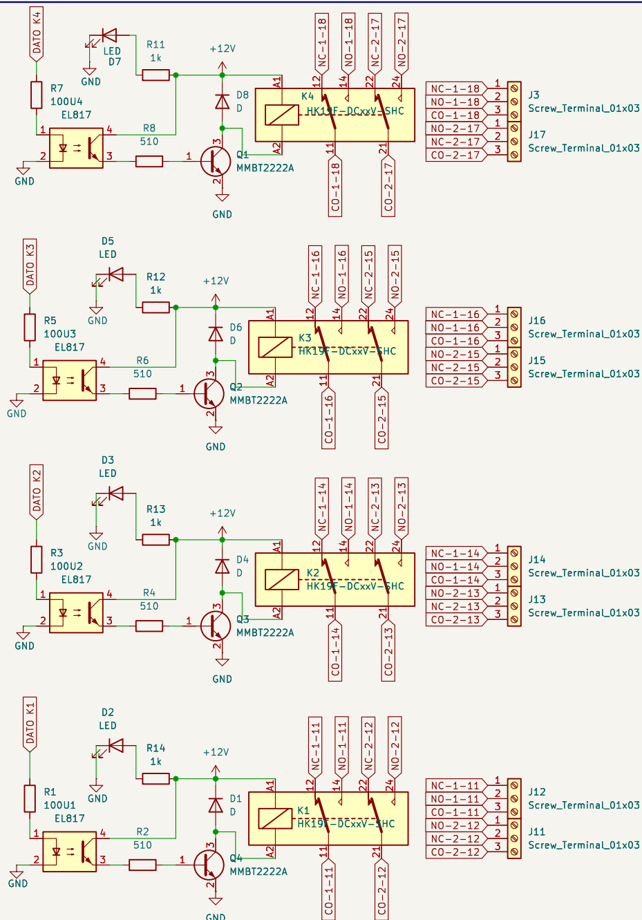
CIRCUITO RELE
