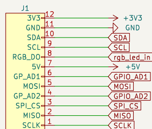
VIK module connector
