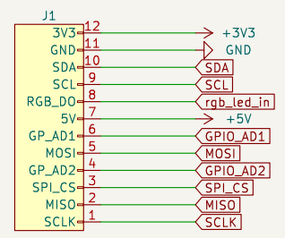
VIK module connector
